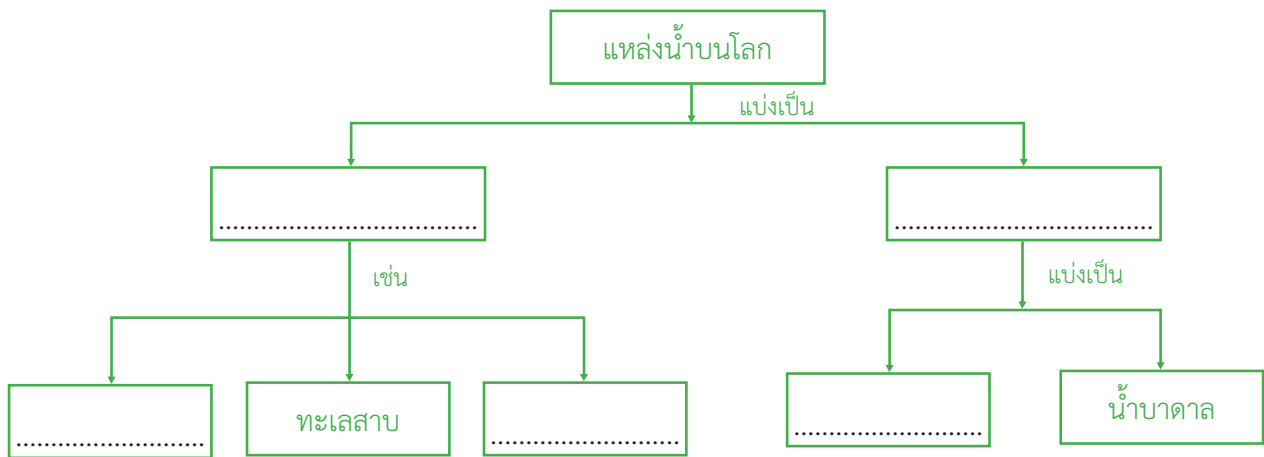
แผนผังแนวคิดแหล่งน้ำบนโลก
