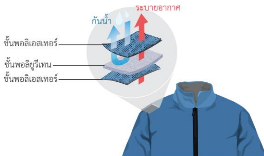
ภาพที่ 4 โครงสร้างของผ้าคอมโพสิต
