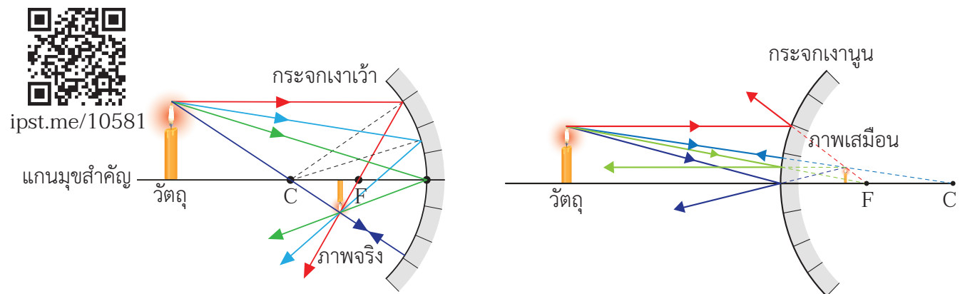
ภาพที่ 3 การเขียนแผนภาพรังสีของแสงเพื่อระบุตำแหน่งของภาพเมื่อวางวัตถุไว้หน้ากระจกเงาโค้ง
