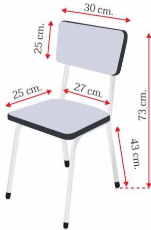
แบบร่างเก้าอี้ แบบที่ 2
